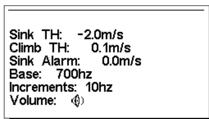
FIGURE 4.21 – Vario acoustique
